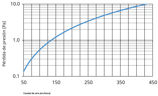
Diámetro: 125 mm / Longitud: 1 m
