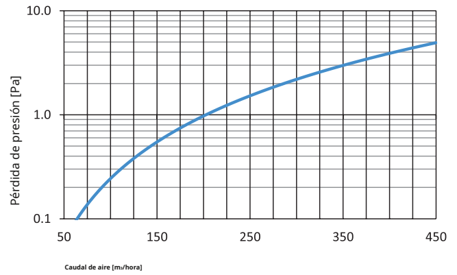
Diámetro: 160 mm / Longitud: 1 m
