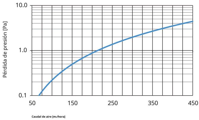
Diámetro: 180 mm
