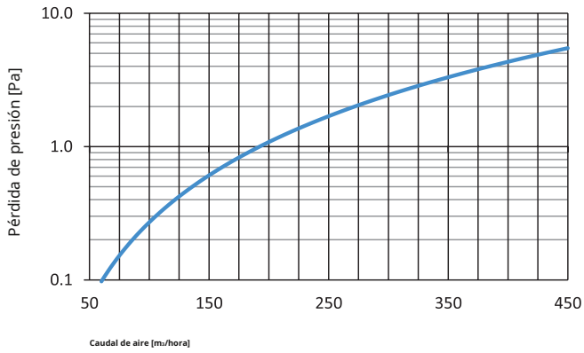
Diámetro: 125 mm
