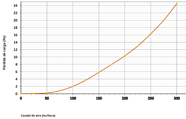
Cuadro de distribución de diagrama de pérdida de carga 8 conectores laterales de difusión Ø125
