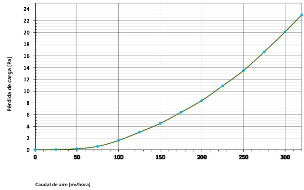
Cuadro de distribución de diagrama de pérdida de carga 8 conectores laterales de difusión Ø160
