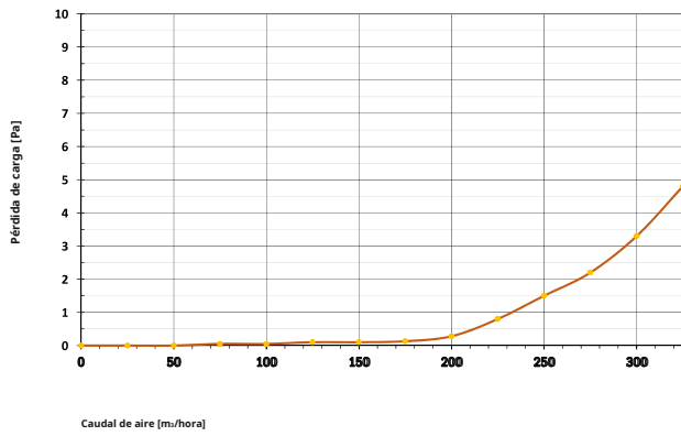
Cuadro de distribución del gráfico de pérdida de carga 12 conectores del lado de difusión Ø160
