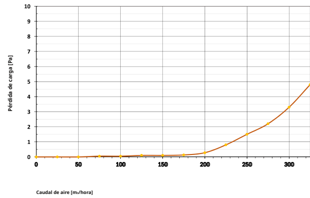
Cuadro de distribución del gráfico de pérdida de carga 12 conectores del lado de difusión Ø180
